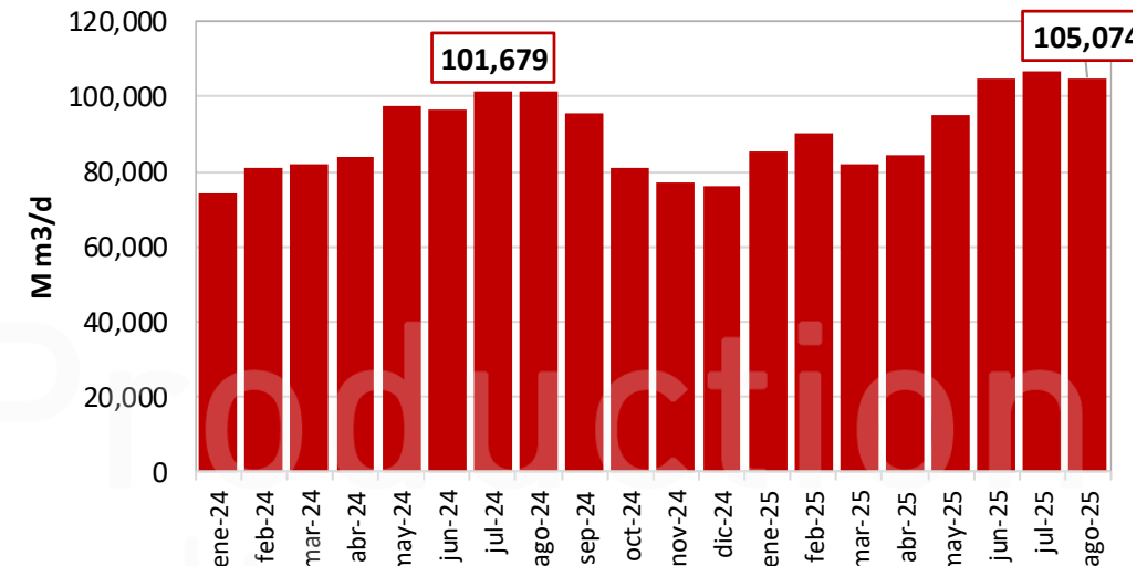
PRODUCCIÓN DE GAS - NOC
