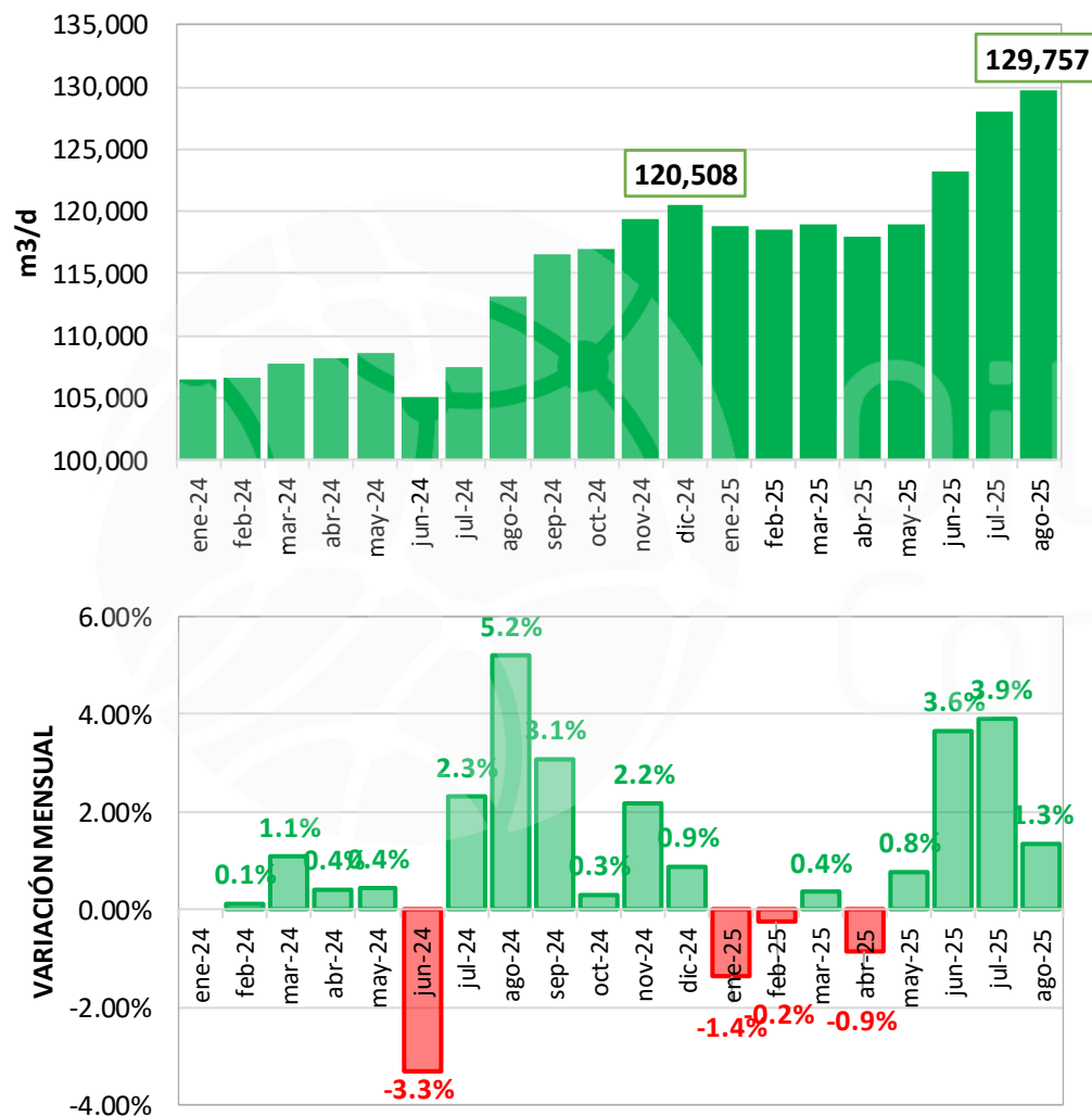
PRODUCCIÓN DE PETRÓLEO
