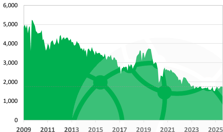
CUENCA AUSTRAL Producción de petróleo - m3/d
