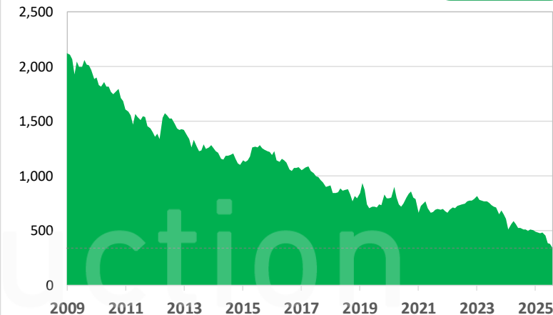
CUENCA NOROESTE Producción de petróleo - m3/d
